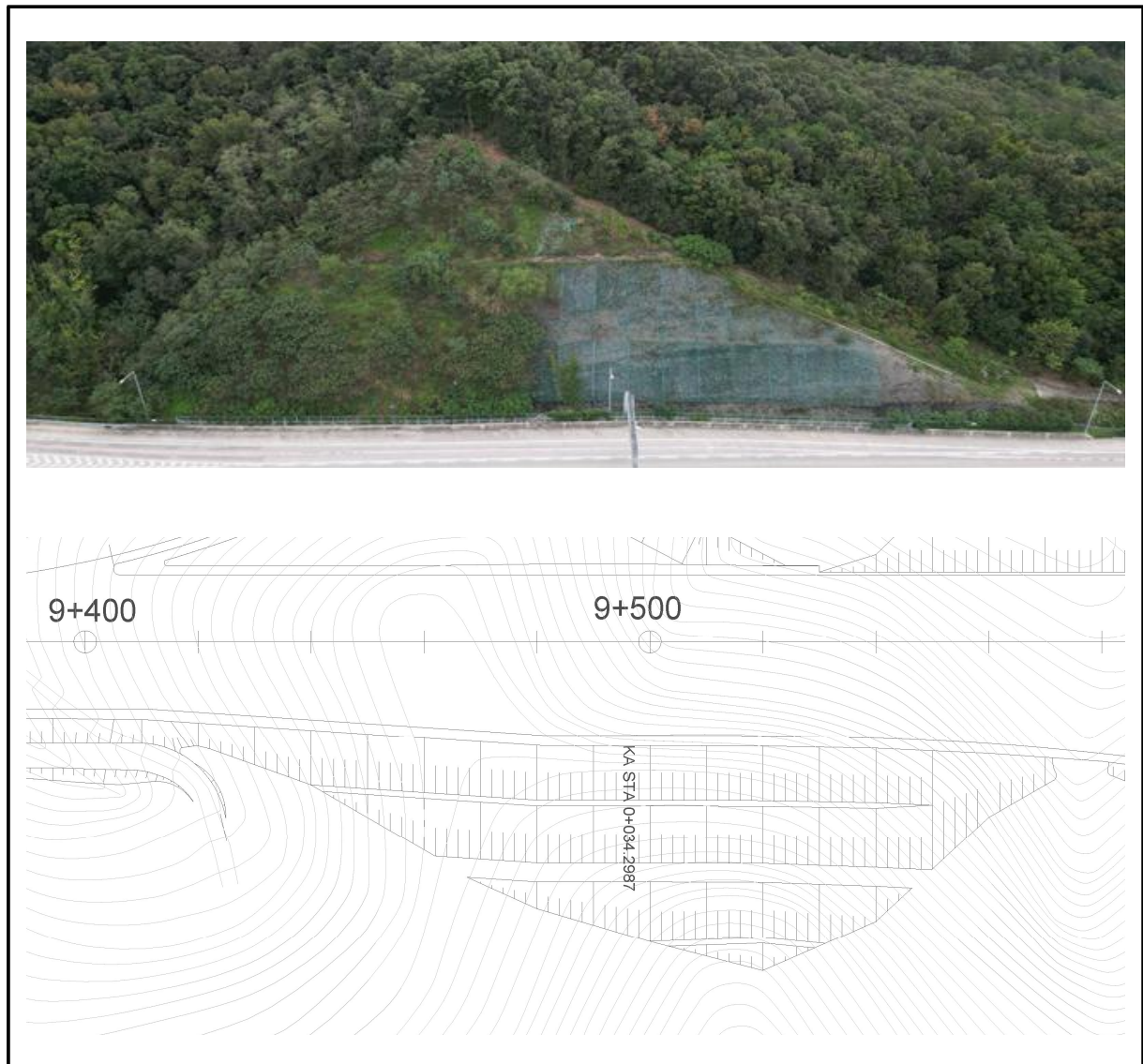
【그림 55.14】 영천절토55 검토대상 비탈면구간
