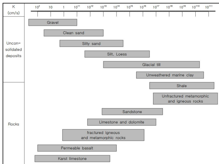
【그림 55.8】 퇴적물 및 암종별 투수계수(Freeze &amp; Cherry, 1979)
