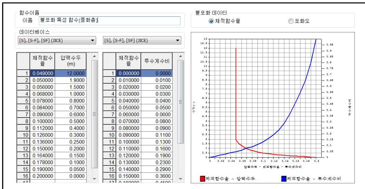
【그림 55.15】 압력수두-체적함수물(포화도)-투수계수비 함수
